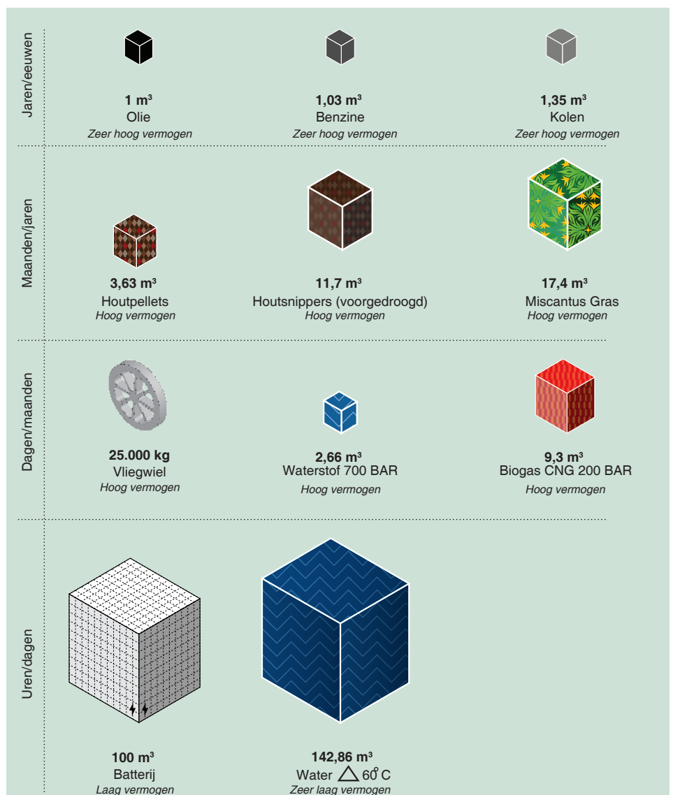
Afb. 14: De karakteristieken van opslagvormen zijn erg uiteenlopend. Naast de dichtheid is het vermogen en de optimale duur van energieopslag verschillend. Batterijen zijn geschikt om korte termijn schommelingen op te vangen, maar hebben een erg laag vermogen en capaciteit. Het kan daarom aantrekkelijk zijn conversieverliezen voor lief te nemen t.b.v. beter hanteerbare opslagvormen, bijvoorbeeld synthetische gasen of waterstof (power 2 gas). Bronnen: Tesla, KWHinzicht.nl, Aqua-cak, NUON, Visionair.nl
