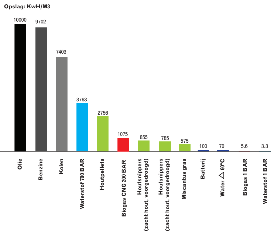
Afb. 8: Opslagdichtheid van verschillende energiedragers (kWh/M 3 )
